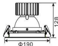
Габаритные размеры
