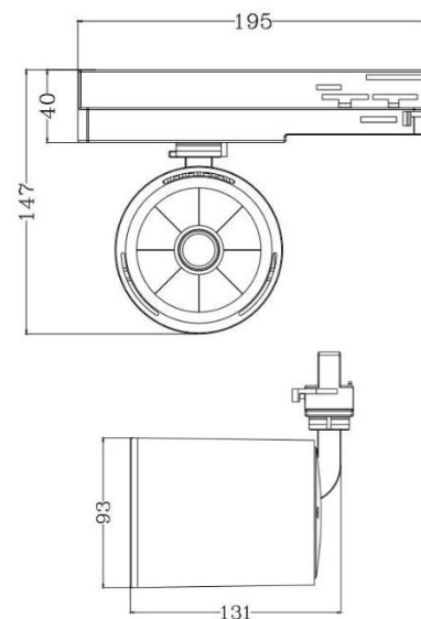
Габаритные размеры
