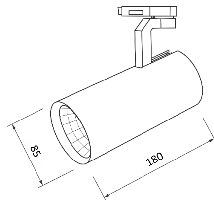
Габаритные размеры
